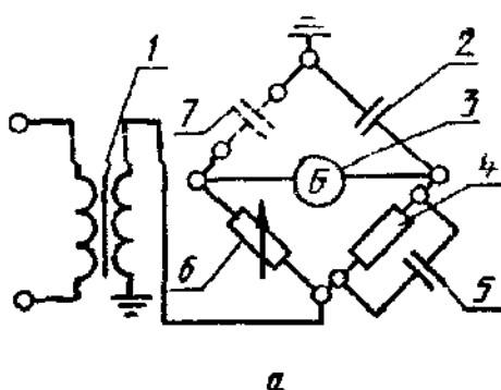
Схема с заземленной диагональю
