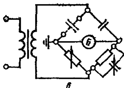
Схема с заземленной диагональю
