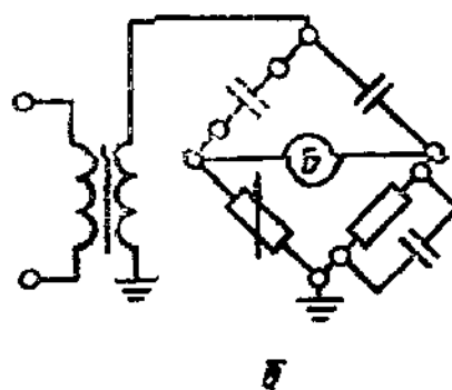
Схема с заземленной диагональю
